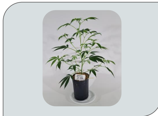
Fórmula B
